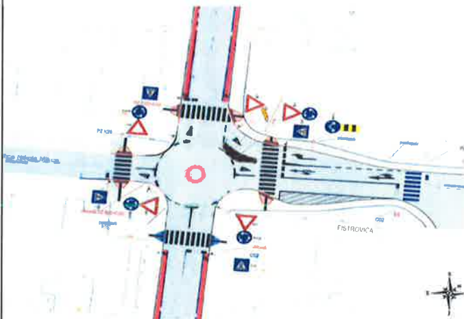
Mini kružno raskrižje Ulica Nikole Šipuća – Nikole Mikca i ceste do Spara
