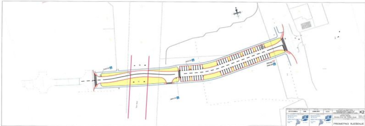
Slika 30 Projekt spajanja Komunalne zone sa Zvonimirovom ulicom
