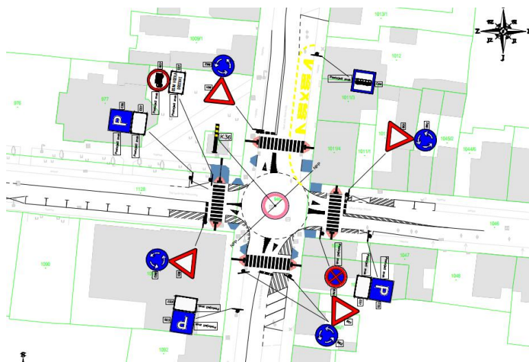
Raskrižje ulica Ante Starčevića - Matije Gupca
