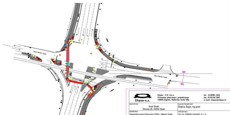
Raskrižje Fistrovićeve - Nikole Tesle
